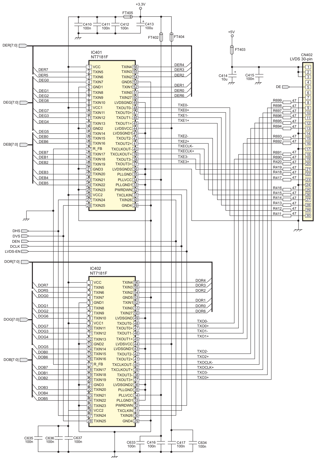
Рис.23 LVDS-интерфейс. Монитор Samsung SyncMaster 172T
